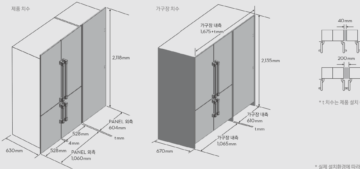
T-TYPE + 컬럼 냉장고 설치했을 때 제품 치수 / 가구장 치수
