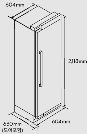
컬럼 냉장과 제품 사이즈
