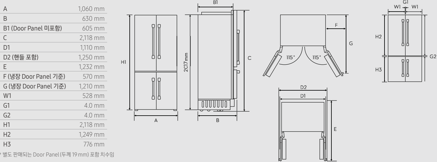
T-TYPE 냉장고 도어 개방 시
