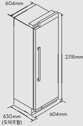
컬럼 냉장고 제품 사이즈
