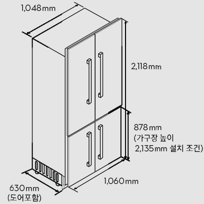
T-TYPE 냉장고 제품 사이즈
