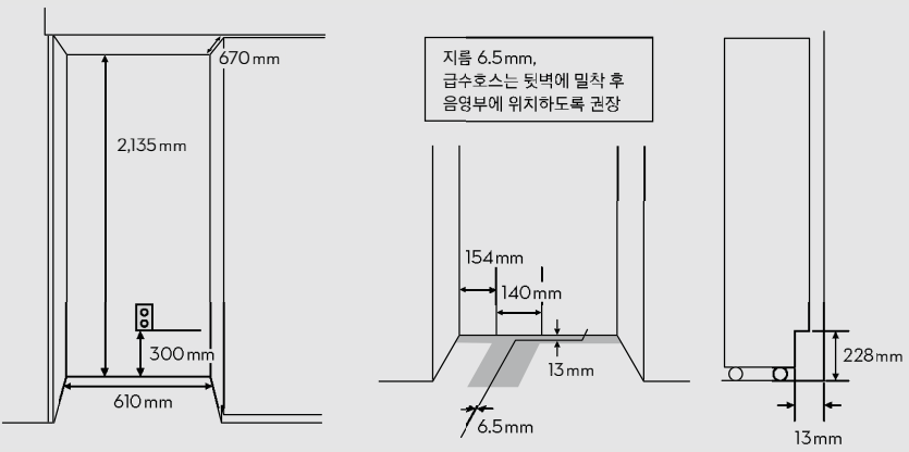
컬럼 냉장고 설치공간
