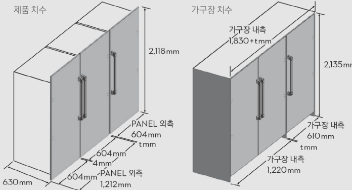
컬럼 냉장과 3대 설치했을 때 제품 치수 / 가구장 치수
