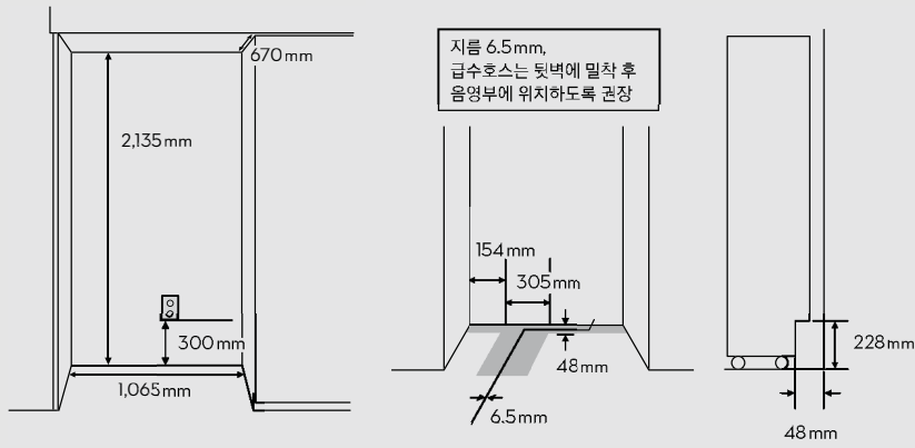
T-TYPE 냉장고 설치공간
