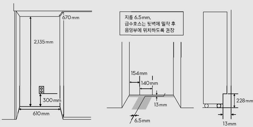
컬럼 냉장과 설치공간
